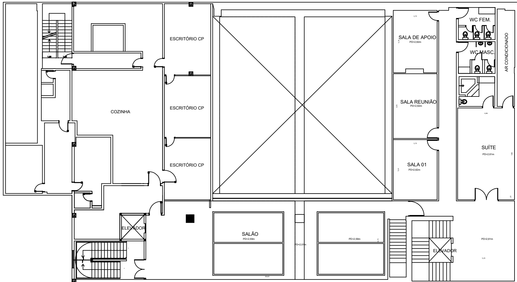
CASA PETRA PLANTA - MEZANINO ESCALA: 1:125
