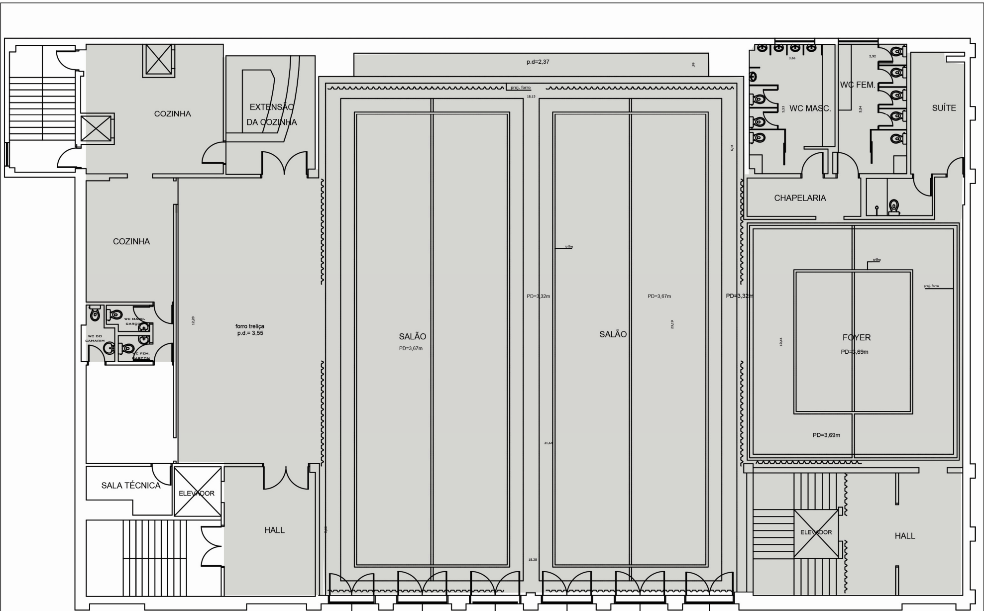
CASA PETRA PLANTA - ATRIO ESCALA: 1:100
