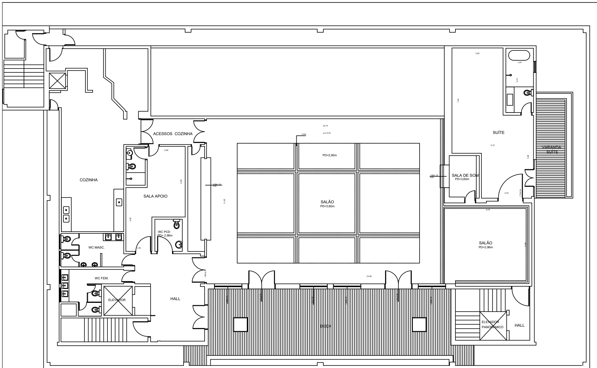
CASA PETRA PLANTA - TERRAÇO ESCALA: 1:100
