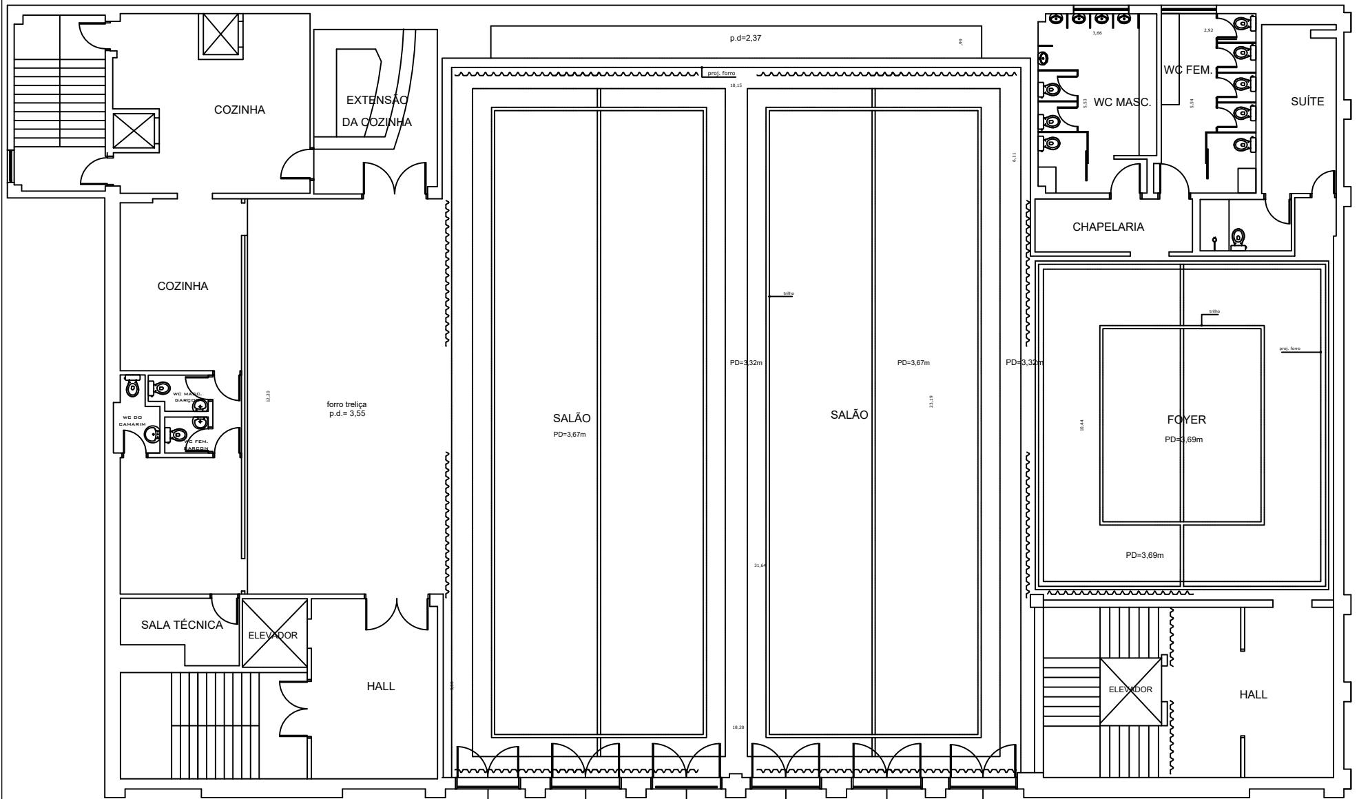
CASA PETRA PLANTA - ATRIO ESCALA: 1:100
